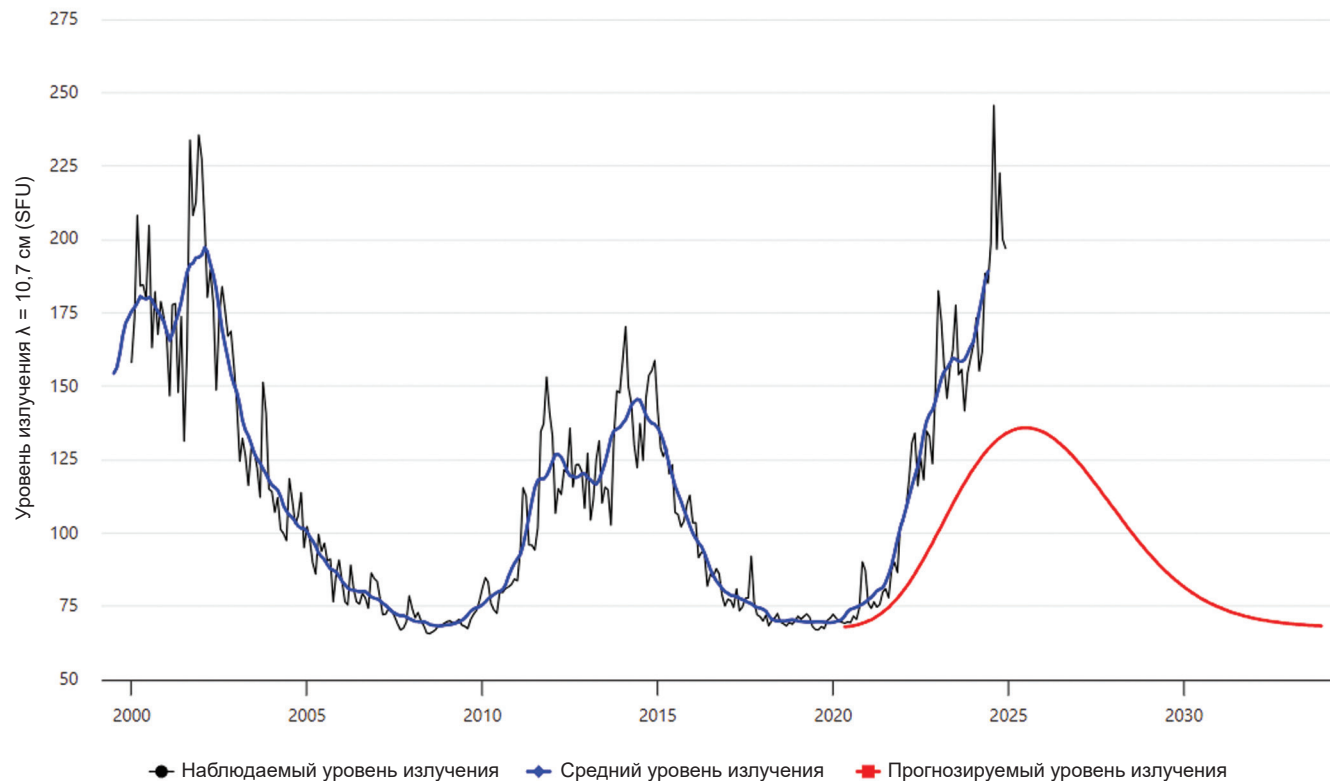
График уровня излучения \lambda = 10,7 см (SFU) в течение солнечного цикла
