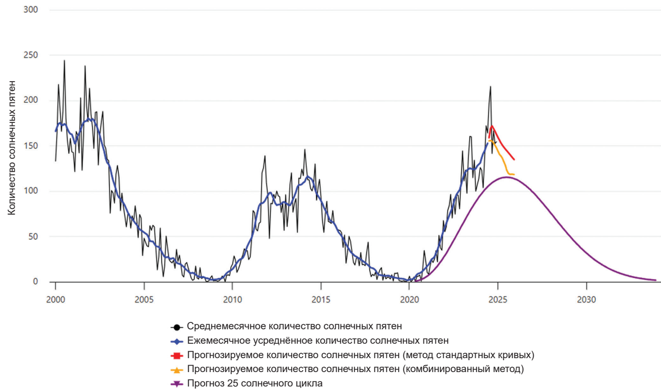
График количества солнечных пятен в течение солнечного цикла
